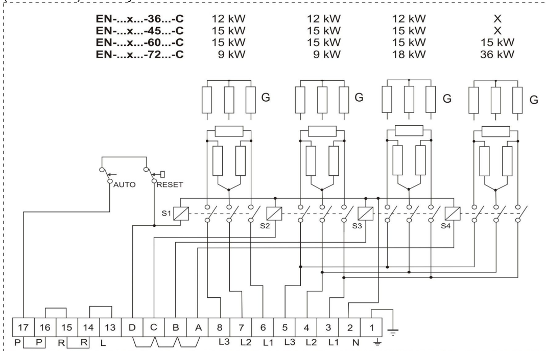
Schemat elektryczny nagrzewnic zasilanych napięciem 400V 3N~. (EN-...-36...-C) dla mocy 36 –72 kW
