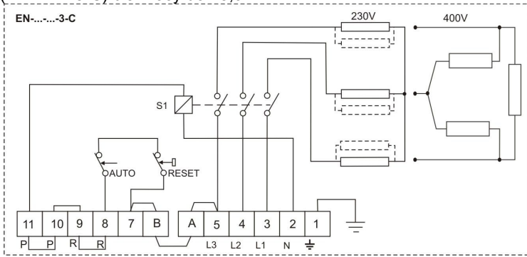
Schemat elektryczny nagrzewnic zasilanych napięciem 400V 3N~. (EN-...-3-C) dla mocy do 15,0 kW
