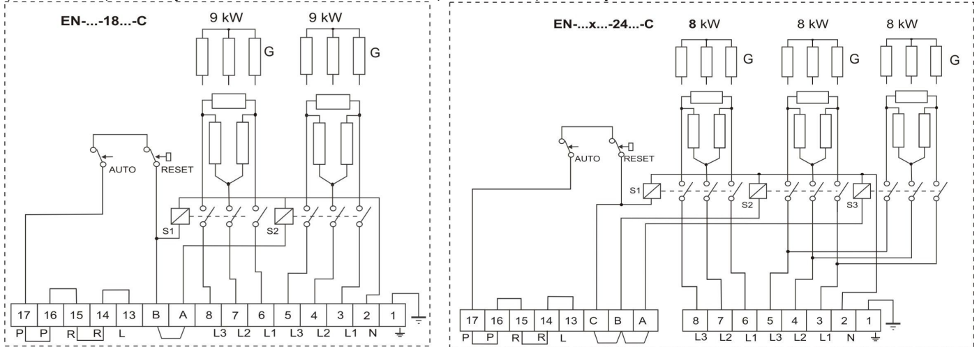
Schemat elektryczny nagrzewnic zasilanych napięciem 400V 3N~. (EN-...-18...-C) dla mocy 18 kW (EN-...-24...-C) dla mocy 24 kW
